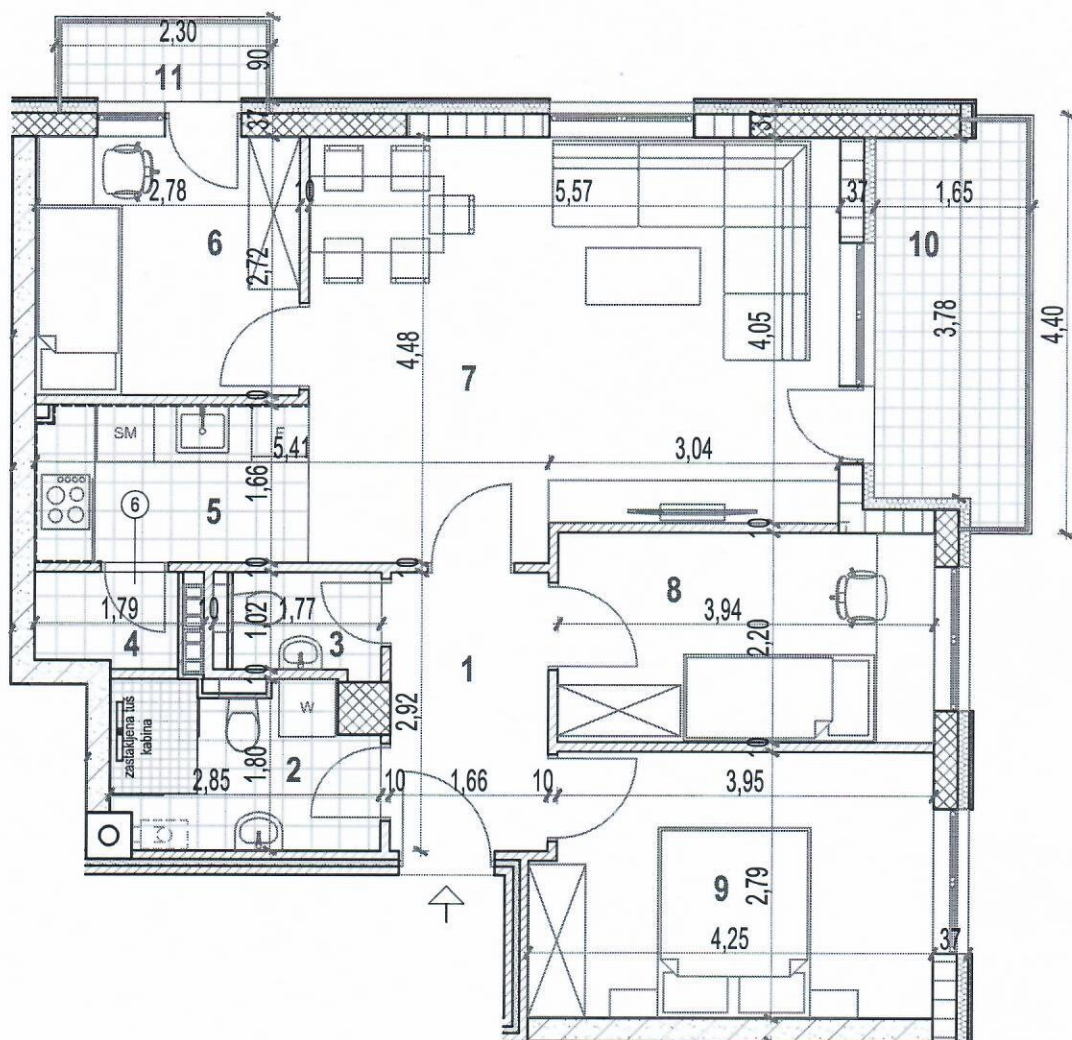
STAN BR. 2,7,12 i 17 - trosoban-ulaz 4
